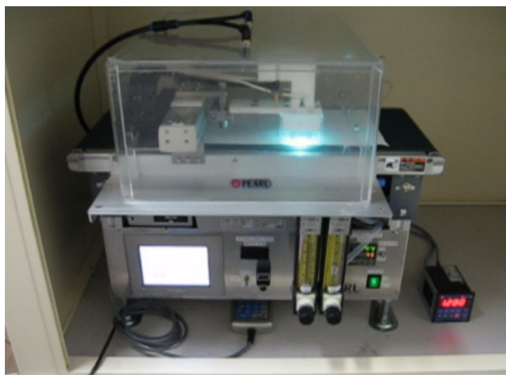
図 1 実験装置概略と写真(装置試作はパール工業㈱による)
